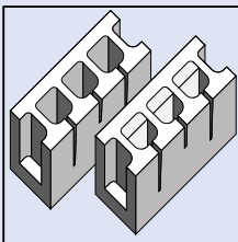
dimensioni modulari cm 20x20x50
