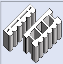
dimensioni modulari cm 12x20x50 (AR12) - 25x20x50 (AR25)
